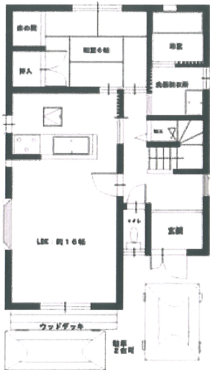
【1階平面図】
